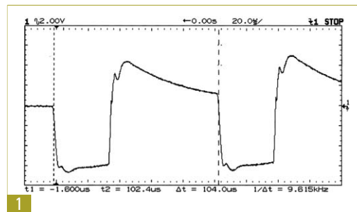
1 KNX-Telegramm
