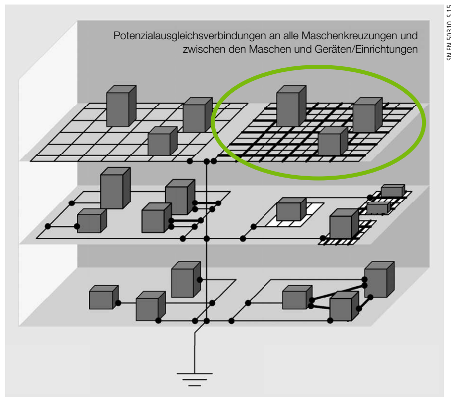
Bild 1 Beispiel von begrenzt ausgelegten Bereichen von Erdernetzwerken in Gebäuden. [1] Prinzipielle Darstellung für die Anwendung z.B. in Serverräumen oder Rechenzentren.
